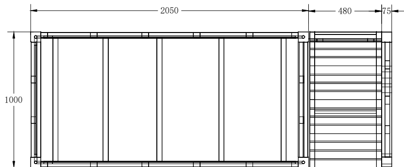
双层木床（2人位步梯） 2605长*1000宽*2250高
