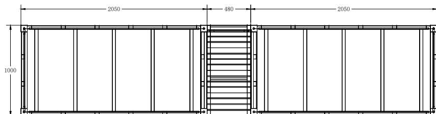
双层木床（4人位步梯） 规格：4580长*1000宽*2250高
